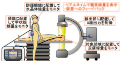
SOF線量計による包括的な放射線量管理システム
